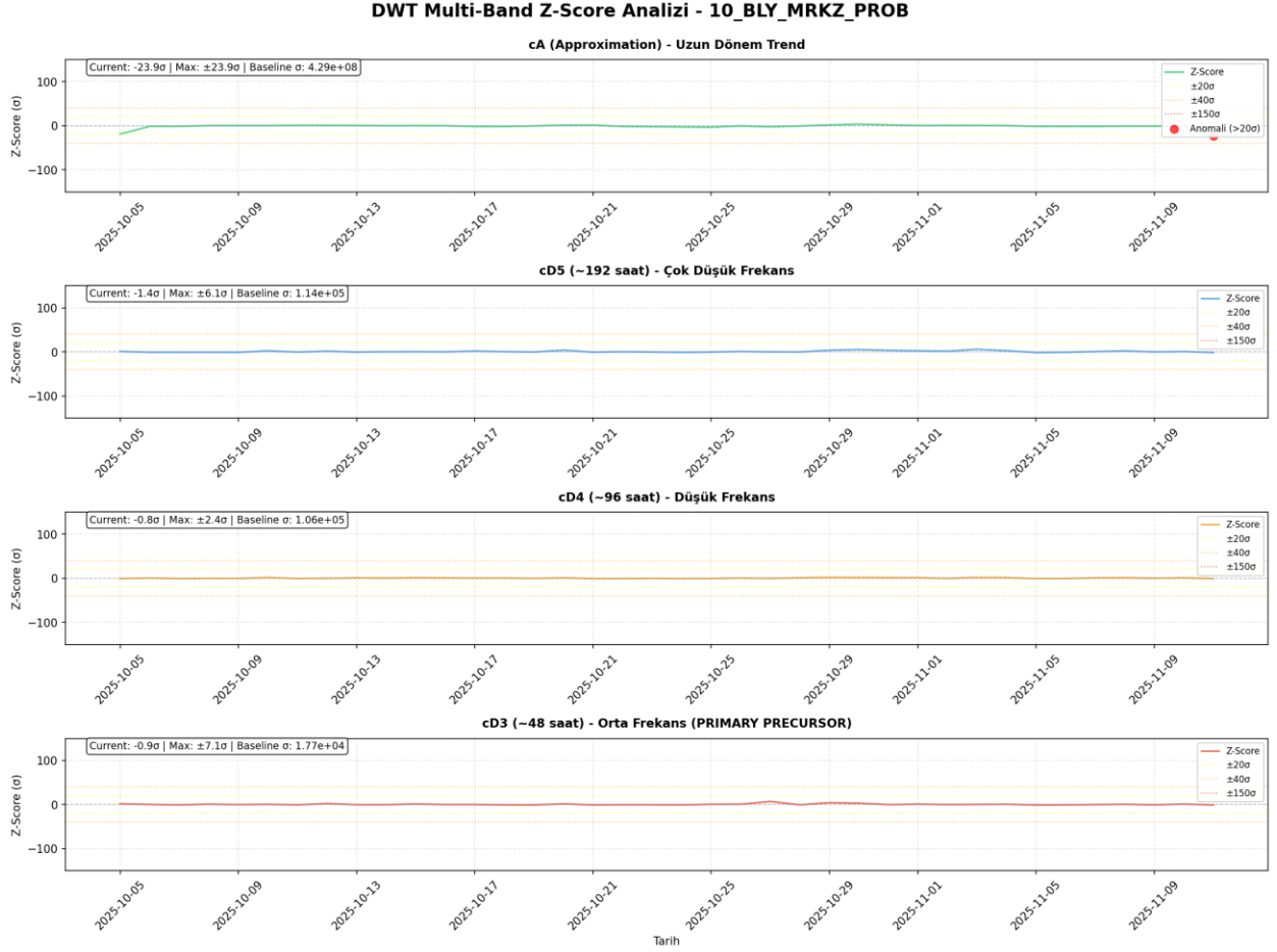
Şekil 15: 10 BLY MRKZ DWT Z-Score analizi.
