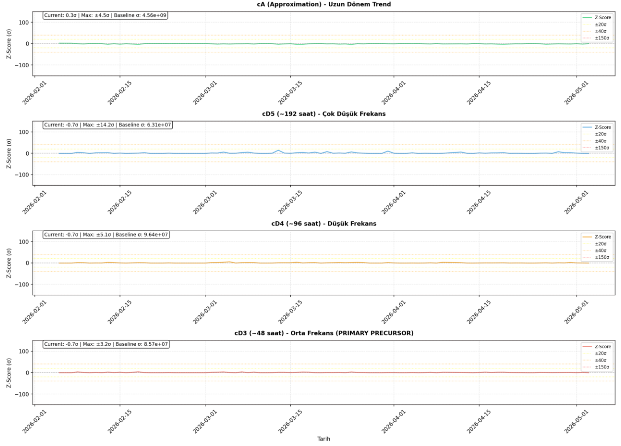
Şekil 18: 10 EDR MRKZ DWT Z-Score analizi.
