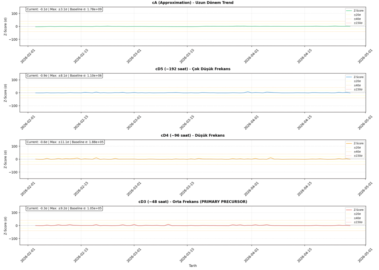
Şekil 21: 10 SIN MRKZ DWT Z-Score analizi.
