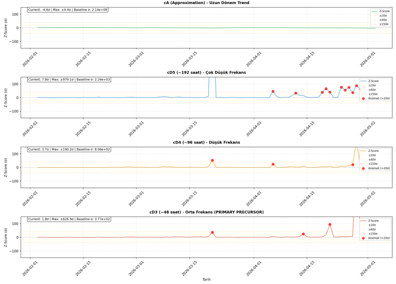
Şekil 19: 10 GNN BLDY DWT Z-Score analizi.
