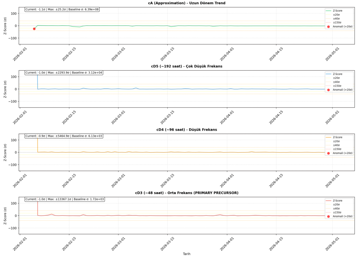
Şekil 17: 10 EDR ALT_N DWT Z-Score analizi.
