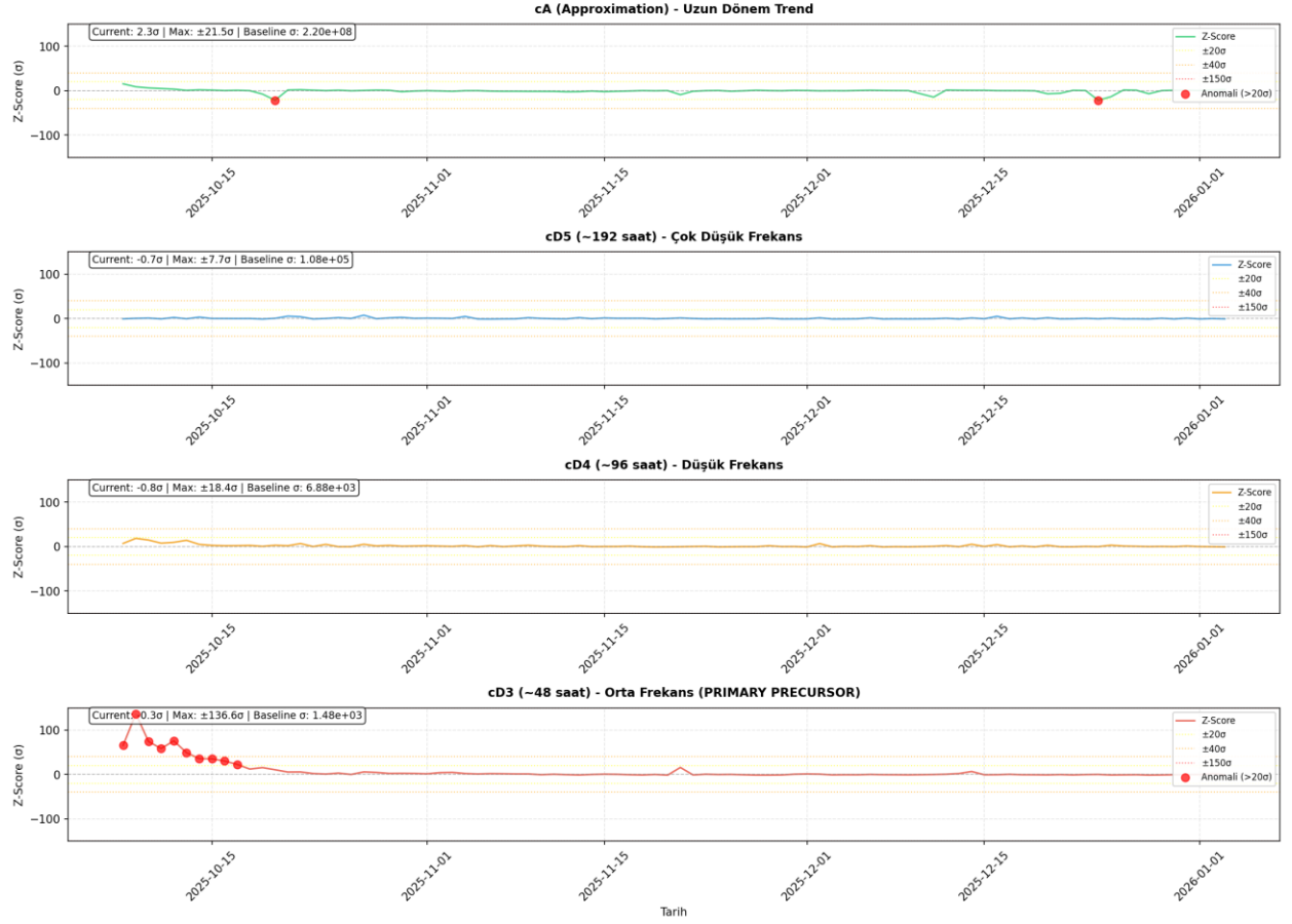
Şekil 16: 10 BSB MRKZ DWT Z-Score analizi.
