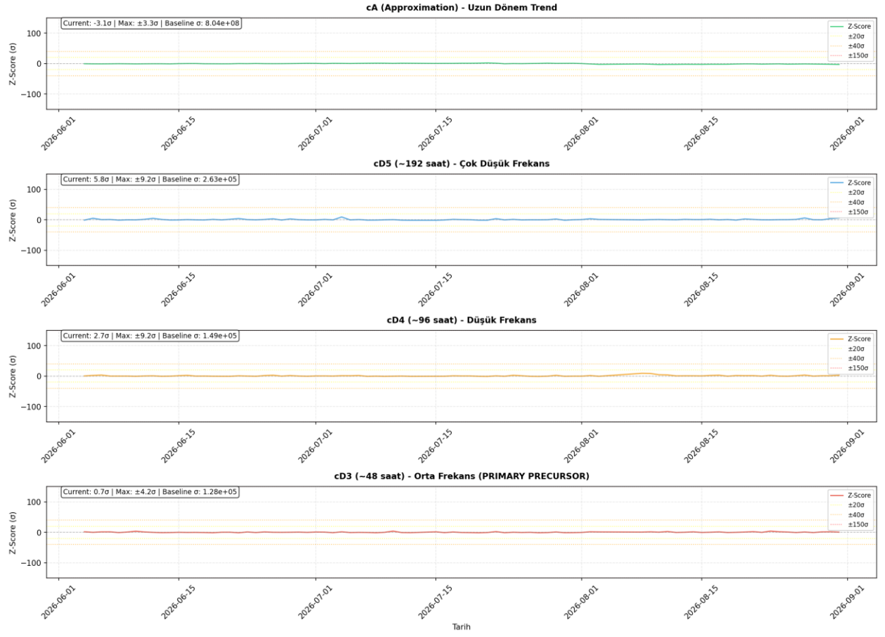
Şekil 21: 10 IVR GKCY DWT Z-Score analizi.
