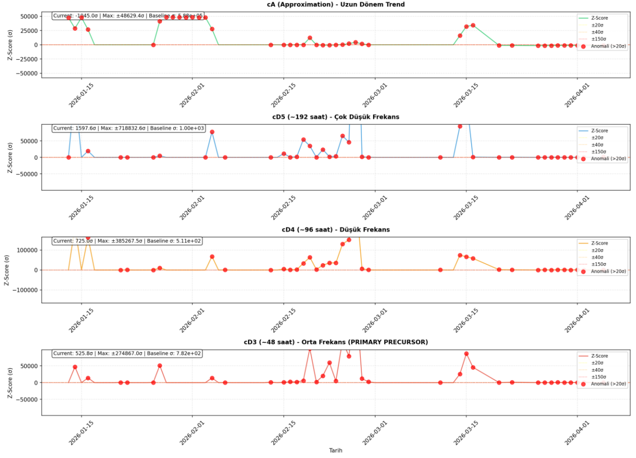
Şekil 22: 10 IVR MRKZ DWT Z-Score analizi.
