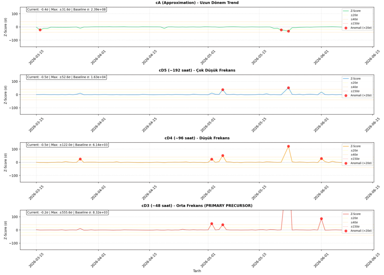
Şekil 23: 10 MAN MRKZ DWT Z-Score analizi.
