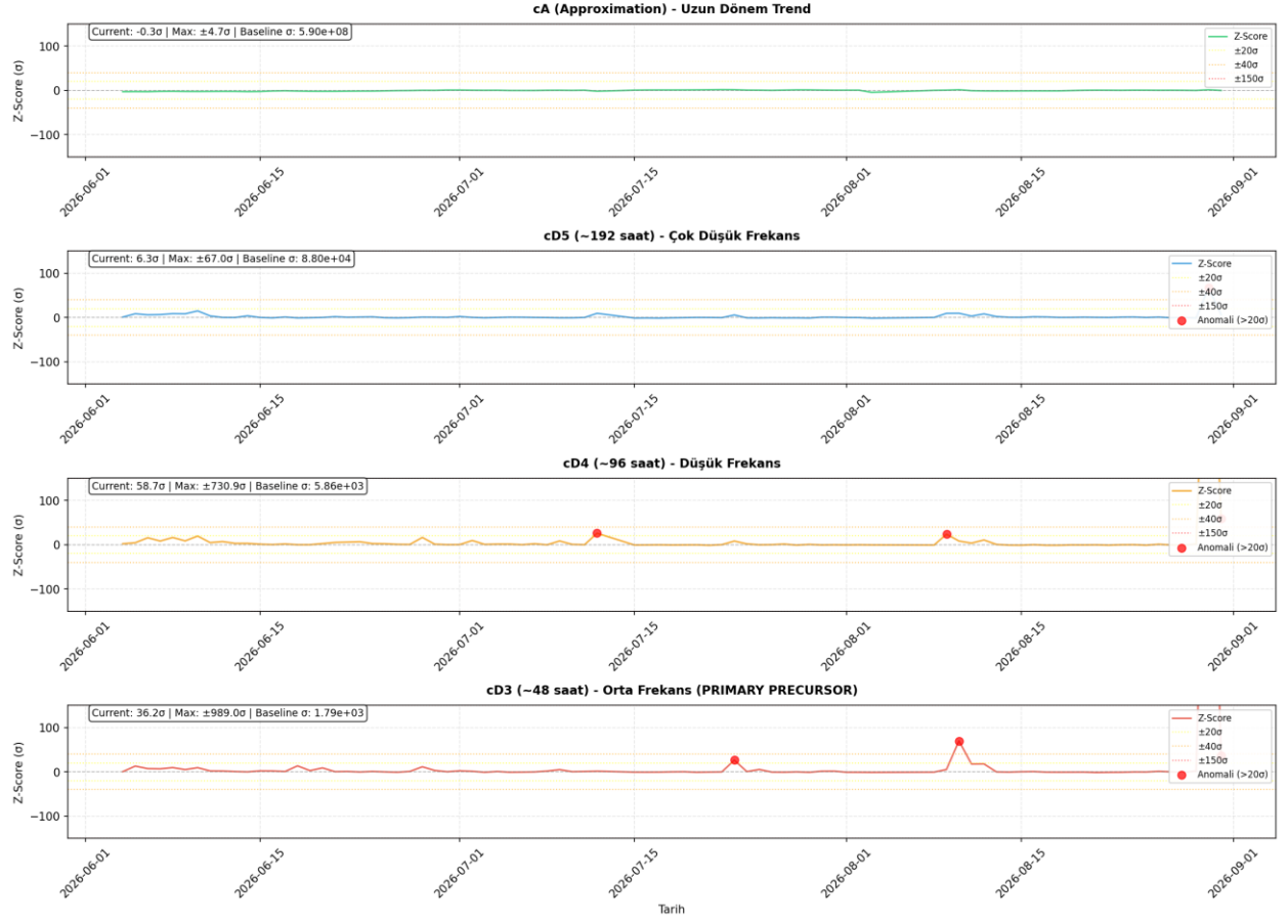
Şekil 24: 10 SIN MRKZ DWT Z-Score analizi.
